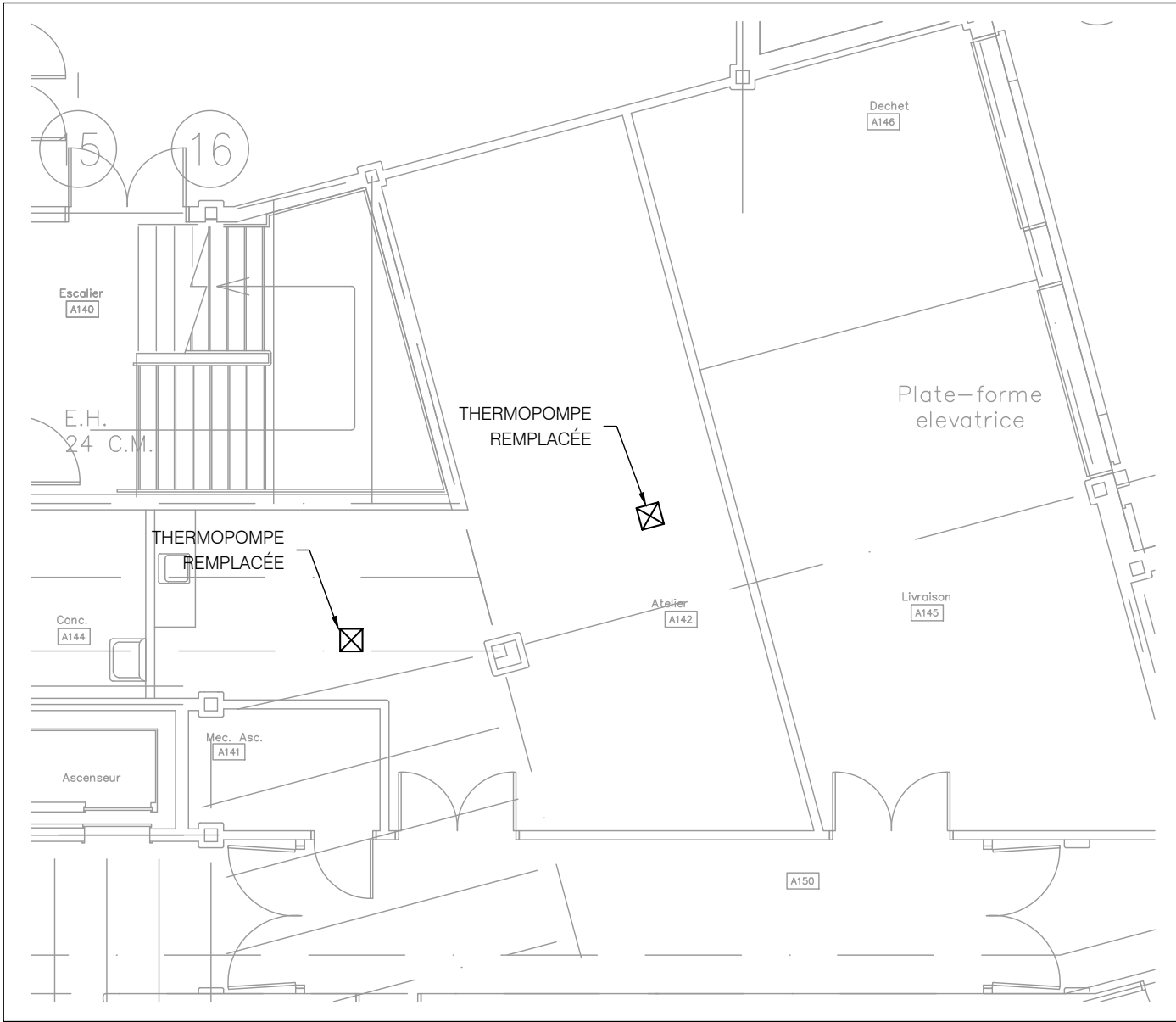
EXTRAIT DU RDC - LOCAL A141 & A142 ÉCH: 1:100 A3 E-101
