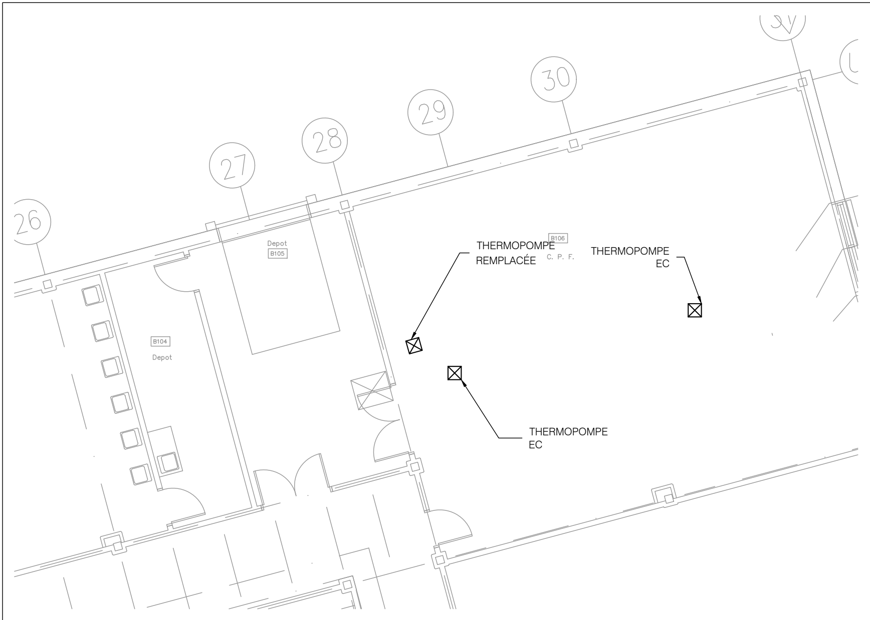
EXTRAIT DU RDC - LOCAL B105 B2 ÉCH: 1:100 E-101
