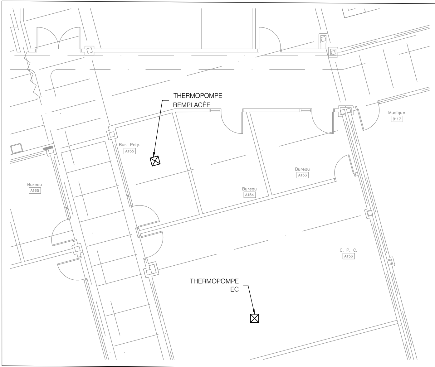
EXTRAIT DU RDC - LOCAL A155 ÉCH: 1:100 A4 E-101
