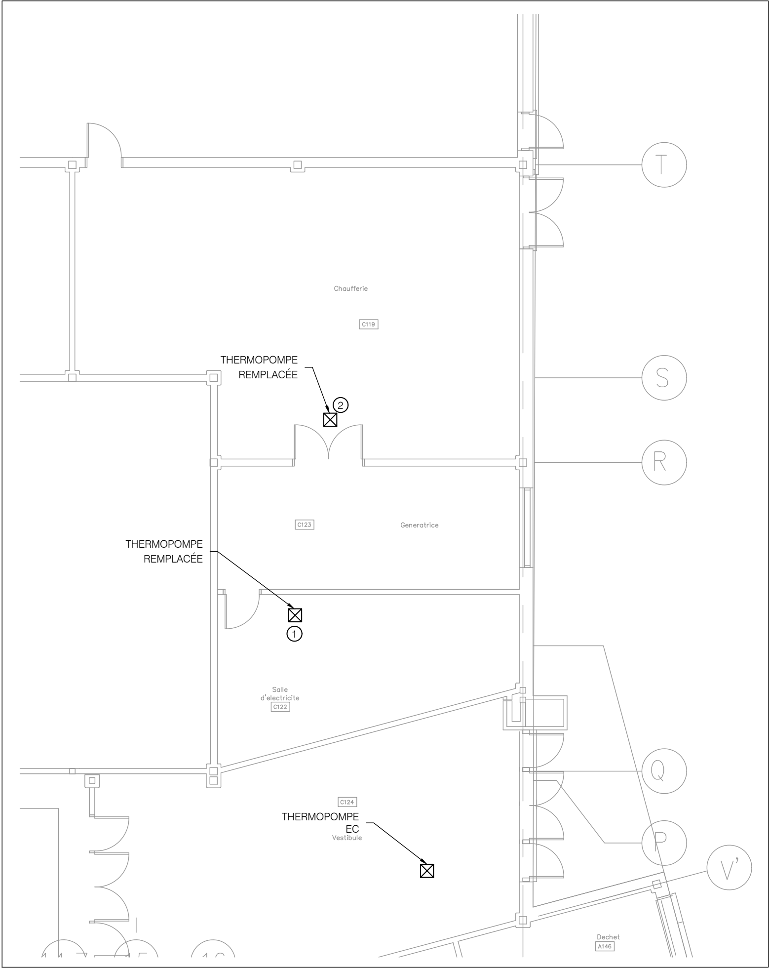
EXTRAIT DU RDC - LOCAL C119 & C122 C3 ÉCH: 1:100 E-101
